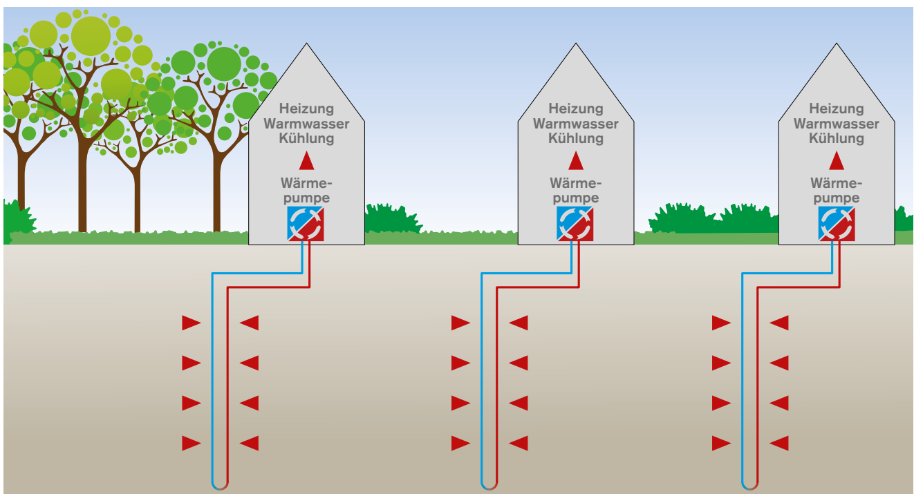
Dezentrale Erdsonden.
